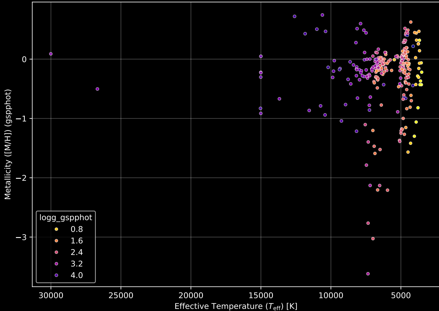
APOGEE DR17 Field: [146+00] Stellar Population Parameters (n= 268)
